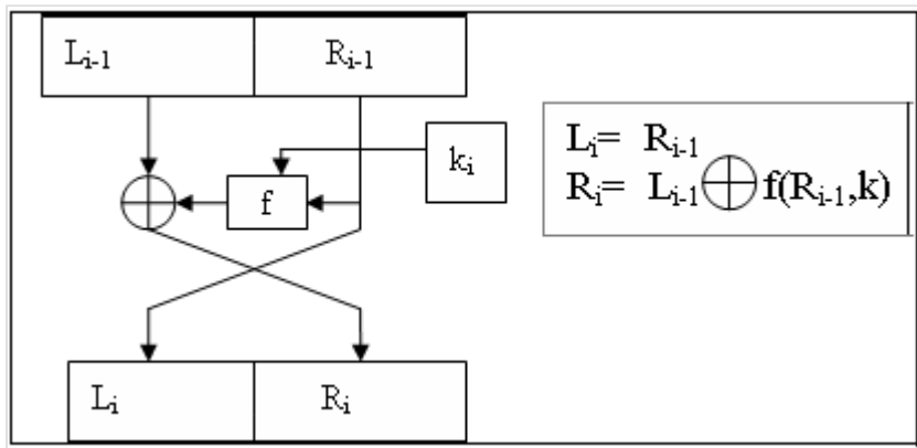
Рис. 1. Прямое преобразование сетью Фейстеля
