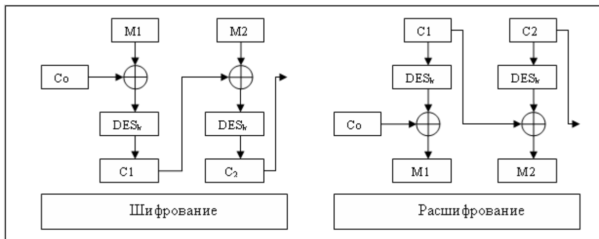
Рис.8 Режим сцепления блоков — CBC
