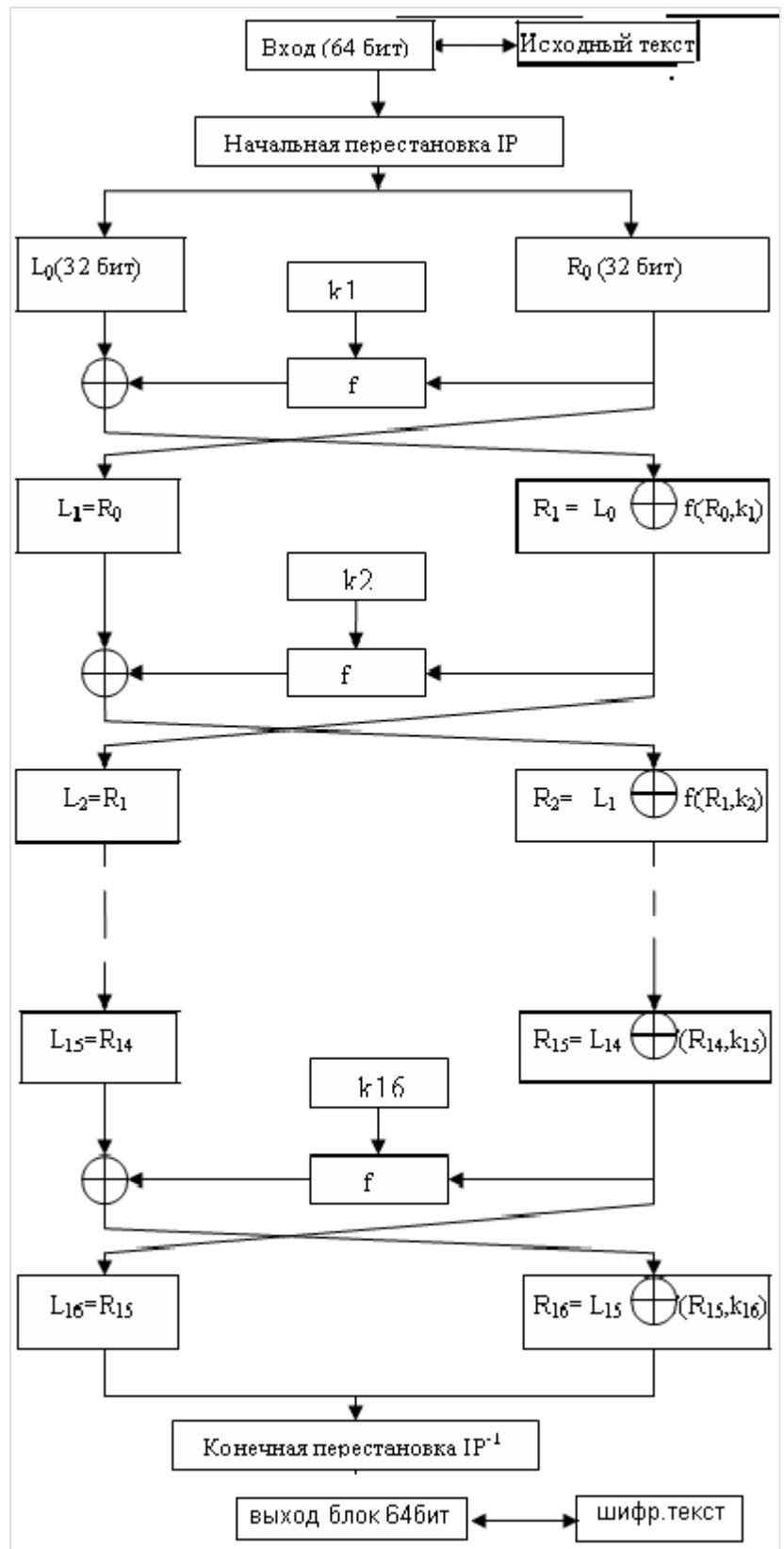
Рис.4 Подробная схема шифрования алгоритма DES
