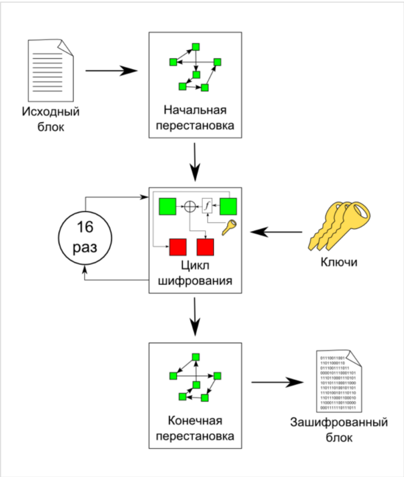
Рис.3 Схема шифрования алгоритма DES
