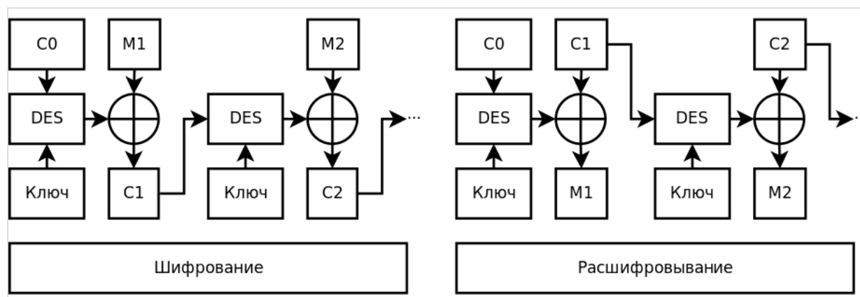
Рис.9 Режим обратной связи по шифротексту — CFB
