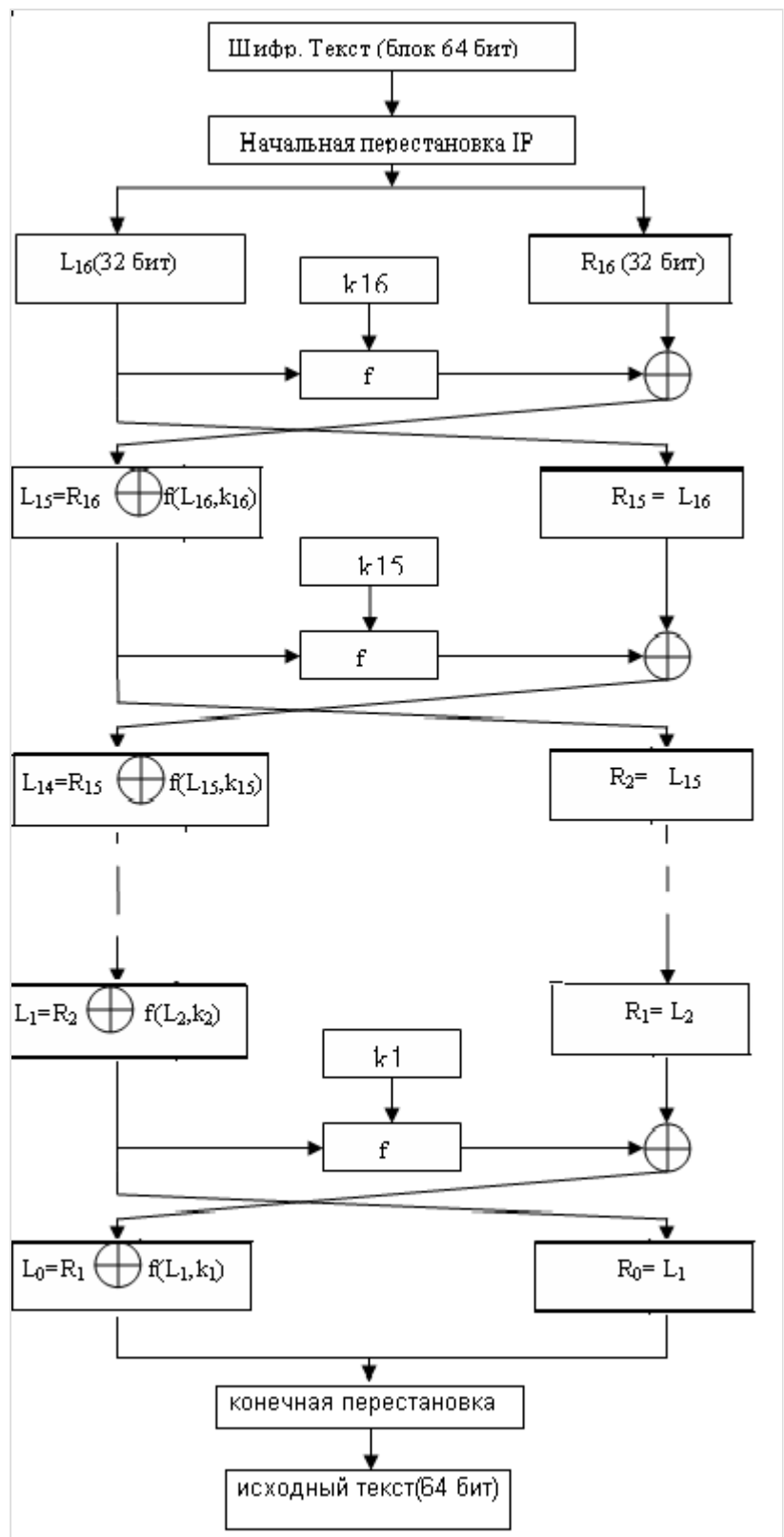
Рис.6 Схема расшифрования алгоритма DES
