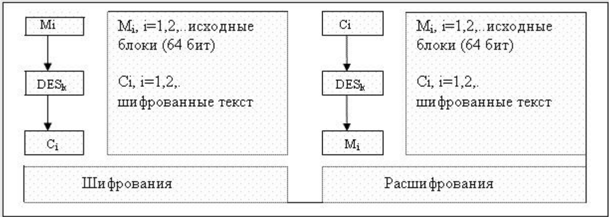
Рис.7 Режим электронной кодовой книги — ECB
