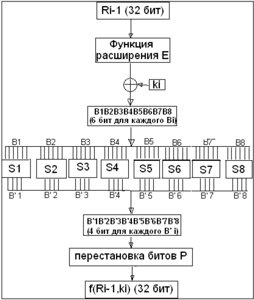
Рис.5 Схема работы функции f
