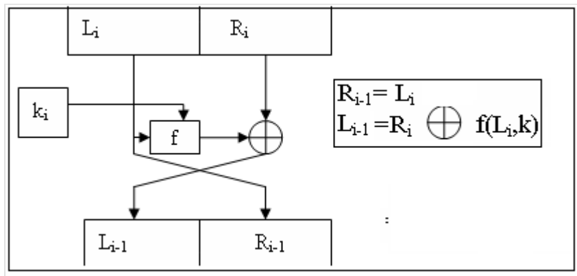
Рис. 2. Обратное преобразование сетью Фейстеля
